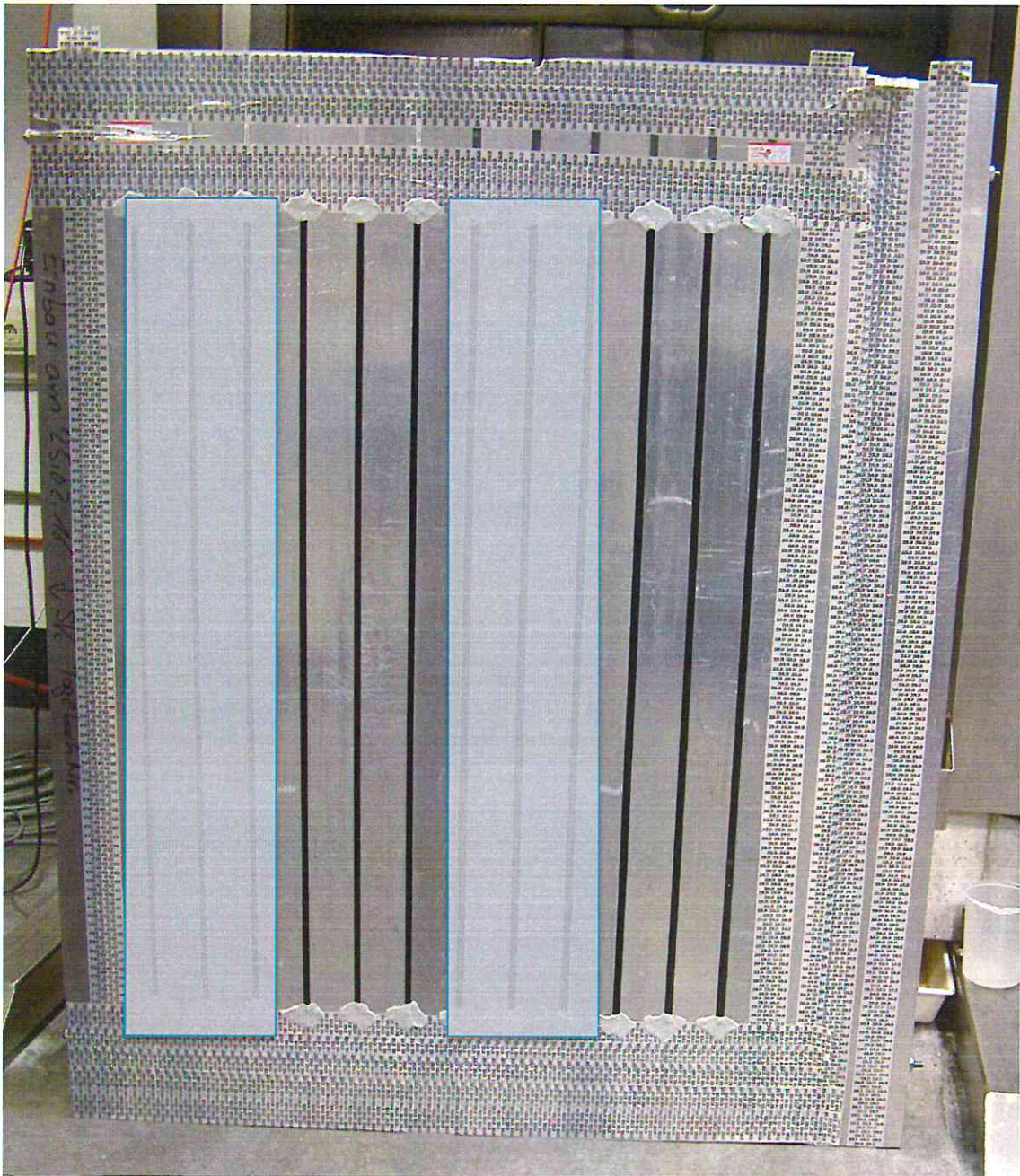
Bild 4: Versuchskörper: mit den eingebauten Fugendichtungsbandern (Blick auf schlagregenbeaufschlagte Seite)
